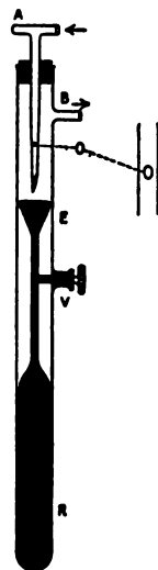
FIG. 45.—Mercury regulator.
