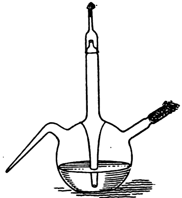
FIG. 415.—Miquel's apparatus.
