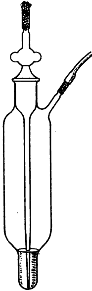
FIG. 414.—Straus and Wurtz' apparatus.
